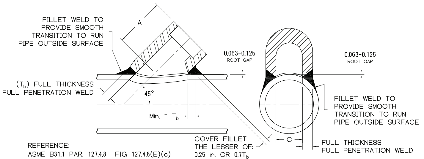
LONGITUDINAL SECTION
